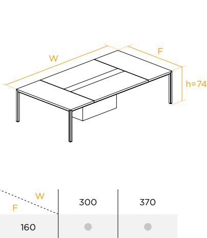
MESAS ENFRENTADAS CON CABECERA FACE-TO-FACE TABLES WITH HEAD TABLE TABLES EN VIS-À-VIS AVEC SÉPARATEUR VERTICAL
