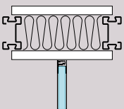
Arranque tabique. Attacco divisorio. Départ cloison.
