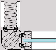
Esquina 90º ciego-vidrio. Angolo 90º opaco- vetro. Coin 90º plein-vitré.
