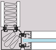
Esquina viva 90º ciego-vidrio. Angolo vivo 90º opaco- vetro. Coin vif 90º plein-vitré.
