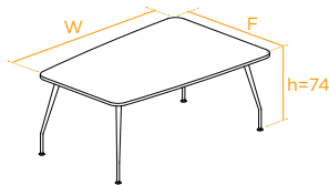
MESA TRAPEZOIDAL T2 T2 TRAPEZOIDAL TABLE TABLE TRAPÉZOÏDALE T2
