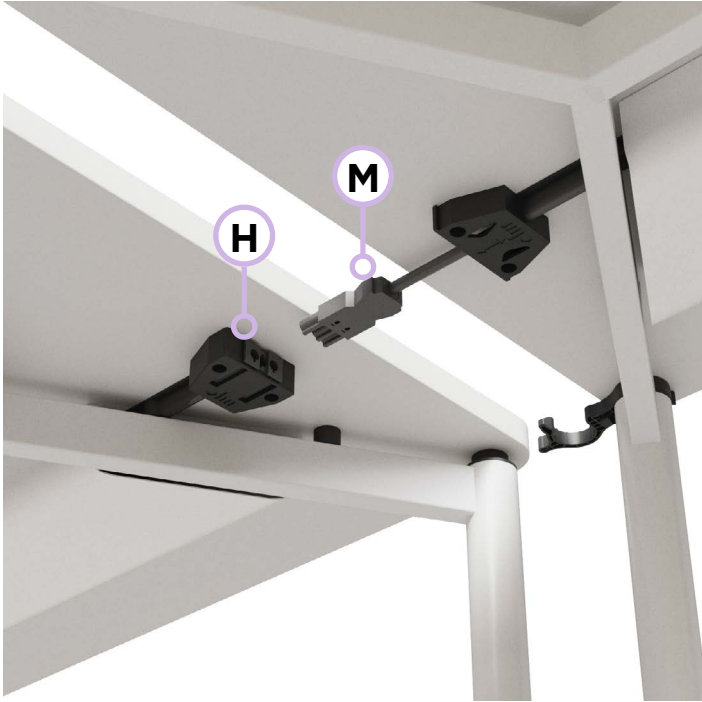
Detalle bajo tablero de la conexión eléctrica entre mesas. Detail of the electrical connection between tables under the work top. Détail sous plateau du raccordement électrique entre tables.
